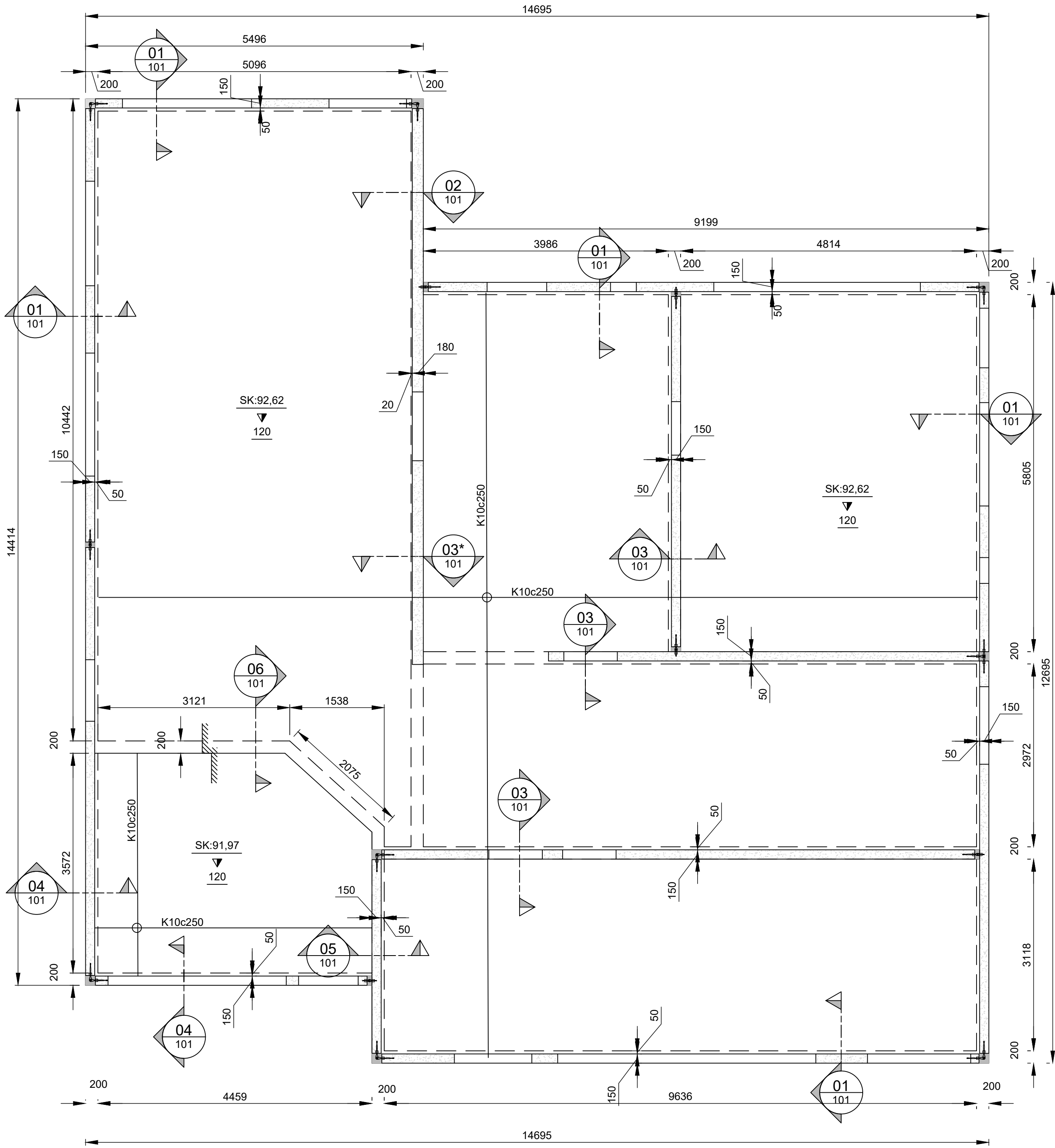
GRUNNMYND MKV. 1:50
